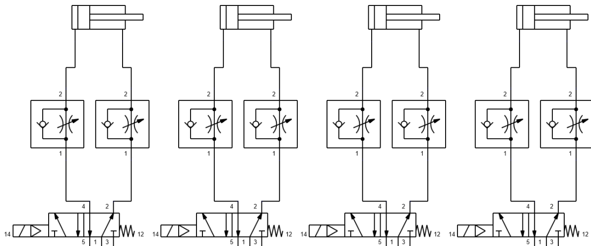
Slika 24. Shema pneumatskog sustava
