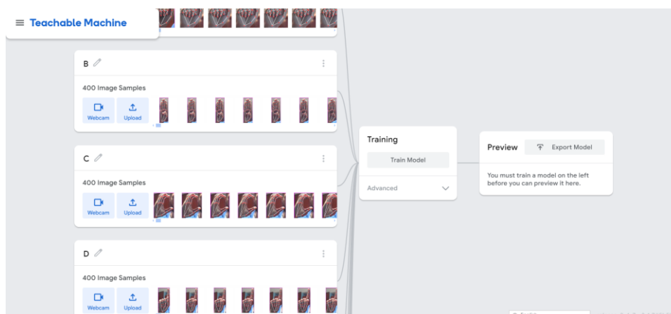
Slika 13. Obuka modela
