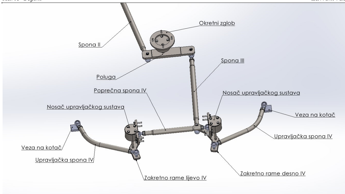
Slika 28. Upravljачki pod sklop IV. osovine sa okretnim zglobo
