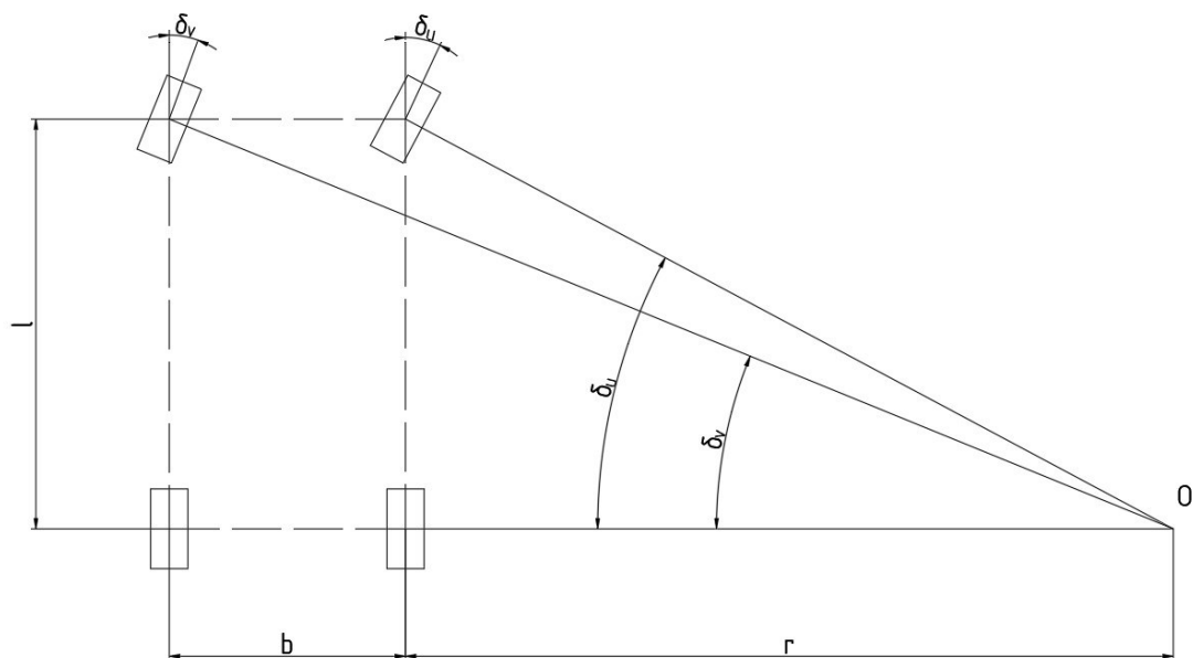
Slika 2. Ackermannova geometrija
