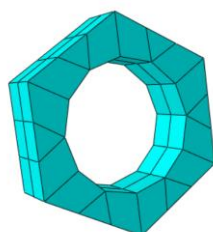
Slika 9. Diskretizacija matice
