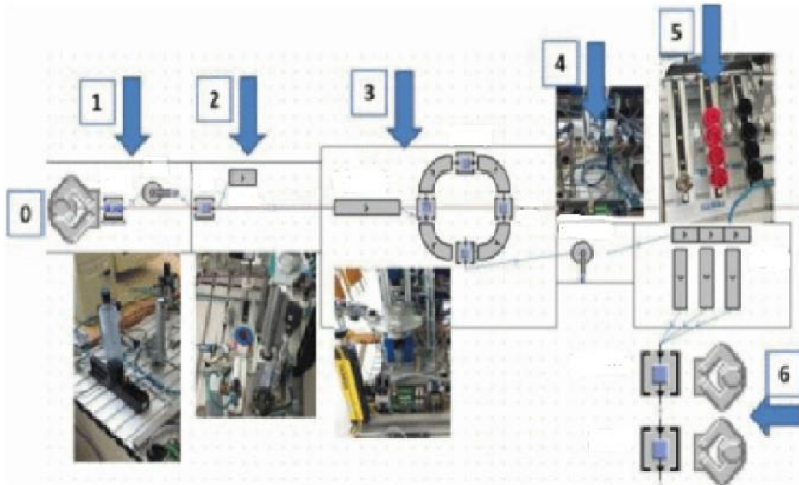
Slika 20. Shema fizičke proizvodne linije [36]
