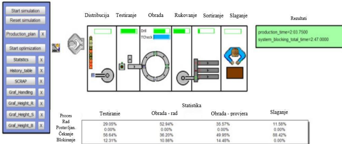
Slika 22. Digitalni blizanac procesa proizvodne linije [36]
