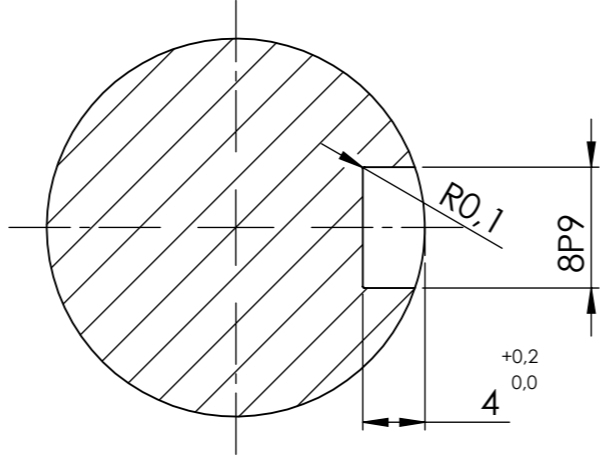
B-B M 2:1
