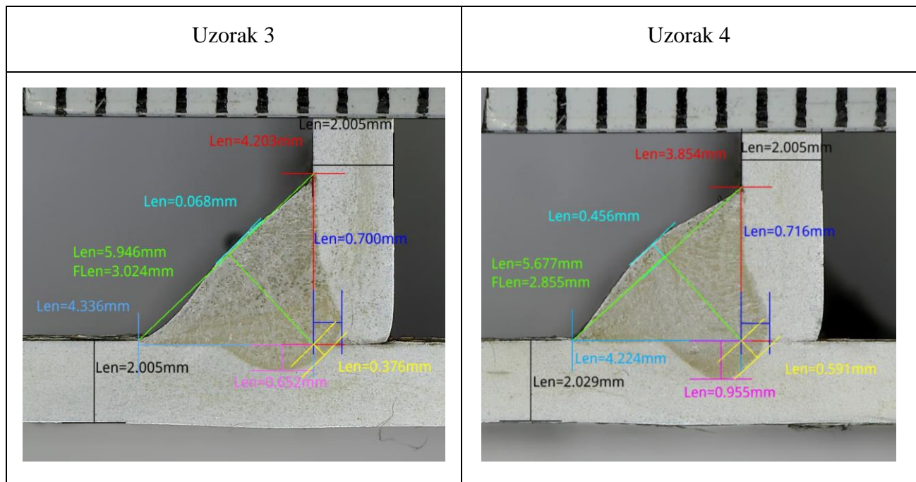
Tablica 18. Makroizbrusci uzoraka 3 i 4 s karakterističnim dimenzijama zavara
