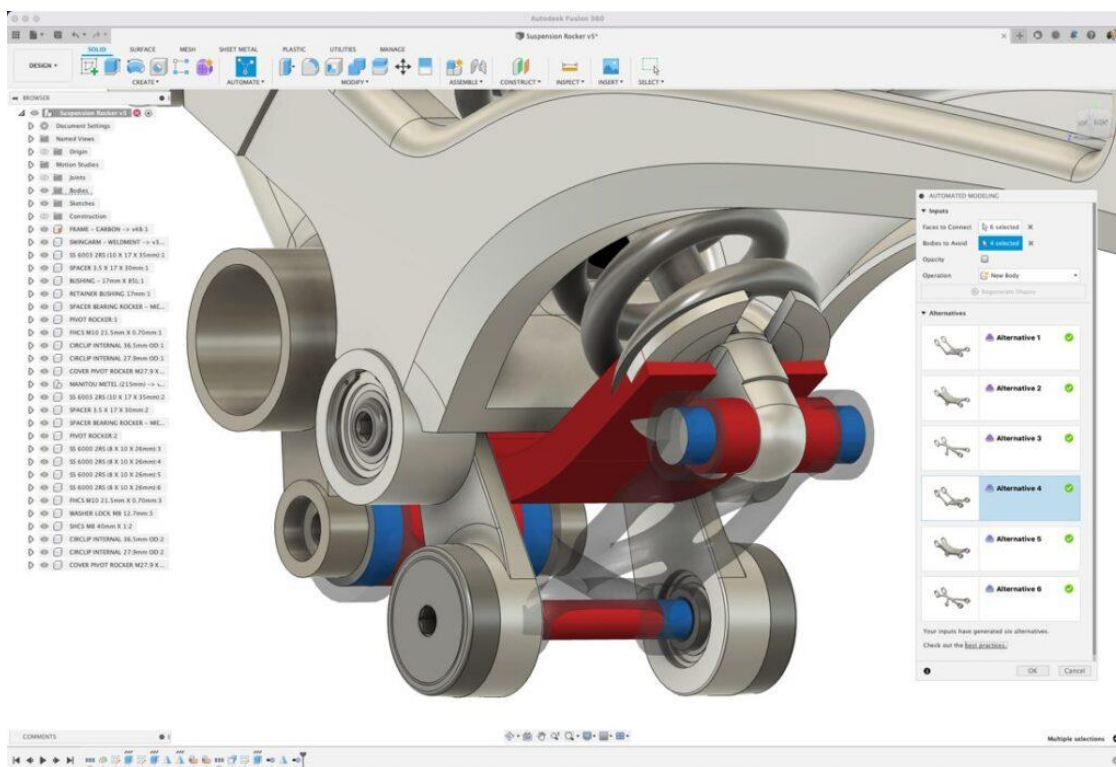
Slika 33. Autodesk Fusion 360 [55]
