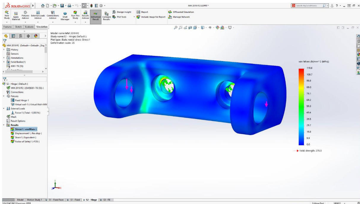
Slika 36. Solidworks Simulation [59]
