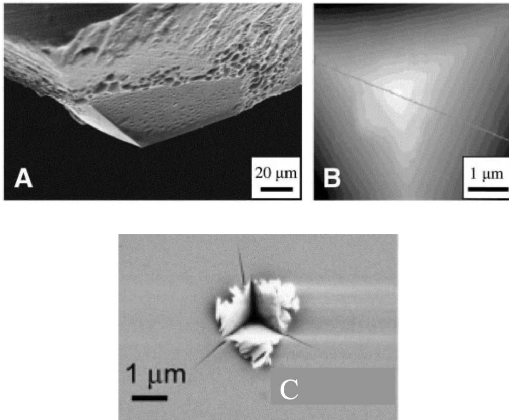
Slika 7. Berkovichev indentor [14]
