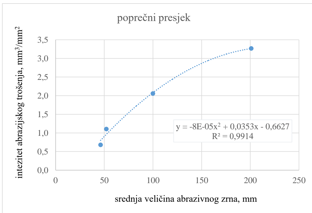
Slika 40. Utjecaj srednje veličine abrazivnog zrna na intenzitet abrazivnog trošenja
