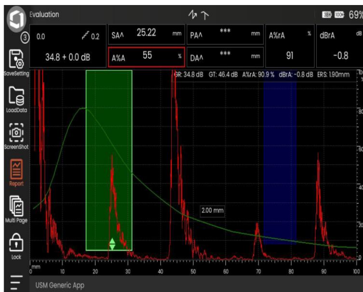
Slika 19. A-prikaz - USM 100 – MB4S – 5 0100
