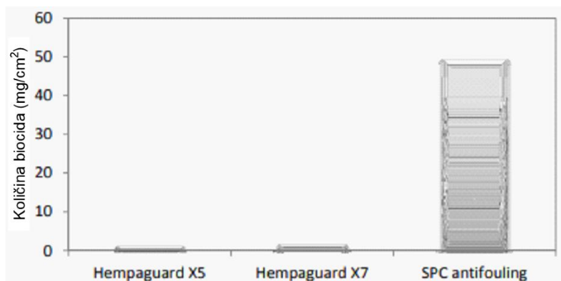
Slika 29. Prosječna količina biocida na cm 2 u HEMPAGUARD X5 i X7 premazima u usporedbi s konvencionalnim SPC premazom (150 µm DSF za HEMPAGUARD i 280 µm DSF za SPC sustav, prema preporučenim vrijednostima) [31]
