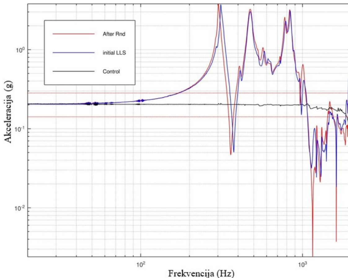
Slika 31. Graf usporedbe LLS prije i poslije, smjer Y
