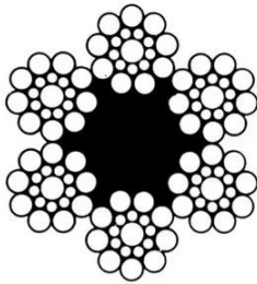
Slika 8. Presjek užeta DIN 3058
