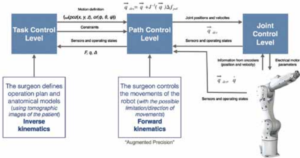
Figure 16. Robot control levels Slika 16. Robotske upravljačke razine
