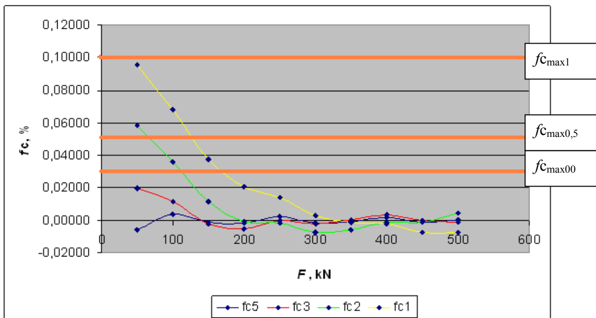
Slika 27: Relativno interpolacijsko odstupanje u ovisnosti o sili za pravac i polinome 2.,3. i 5. stupnja za etalon Z4/500 kN
