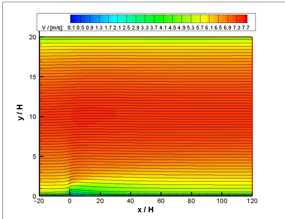
Slika 6.49 Prepreka J – Polje apsolutne vrijednosti brzine
