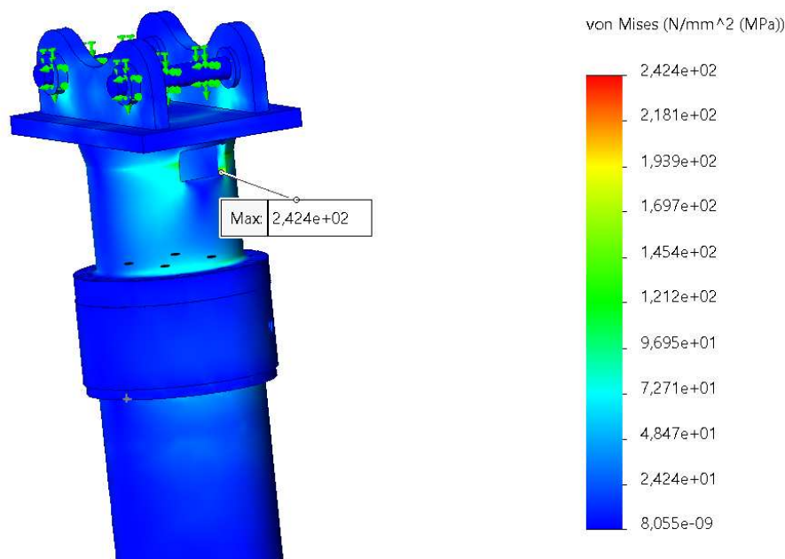
Slika 65. Napreznje konstrukcije
