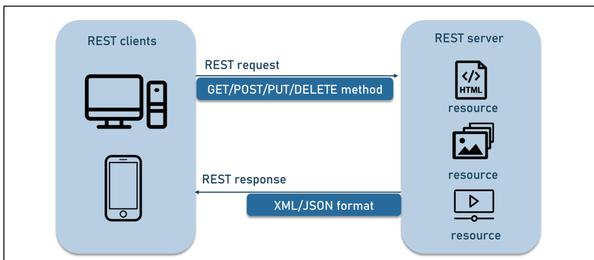
Slika 17 Shematski prikaz načina rada REST API-ja [35]
