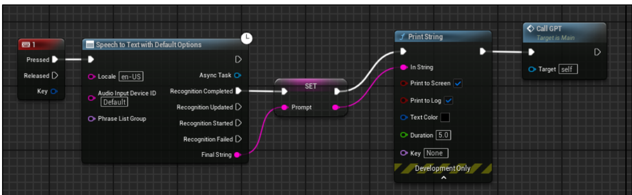
Slika 38 Funkcija za pretvaranje govora u tekst i poziv funkcije „Call GPT“
