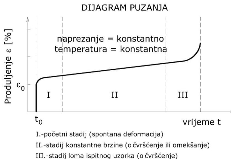
Slika 7. Dijagram puzanja [5]
