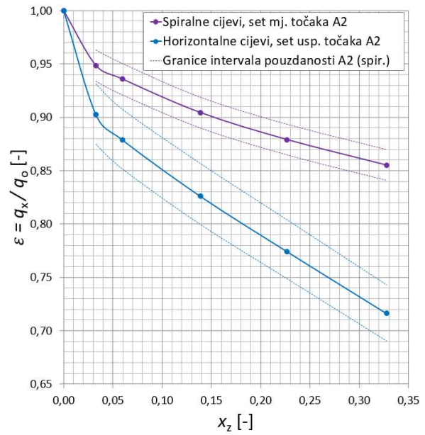
Slika 74. Usporedba negativnih utjecaja kod spiralnih i horizontalnih cijevi u setu točkaka A2
