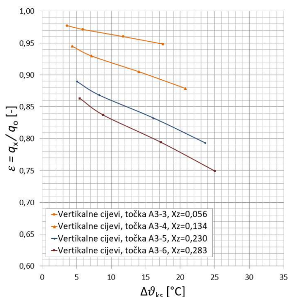
Slika 45. Ovisnost parametra \varepsilon o temp. potencijalu u setu usp. točaka A3 (vertikalne cijevi)
