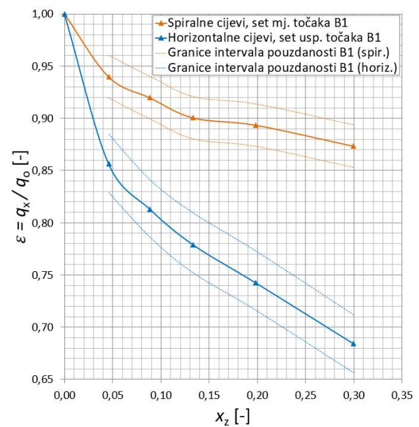
Slika 76. Usporedba negativnih utjecaja kod spiralnih i horizontalnih cijevi u setu točkaka B1
