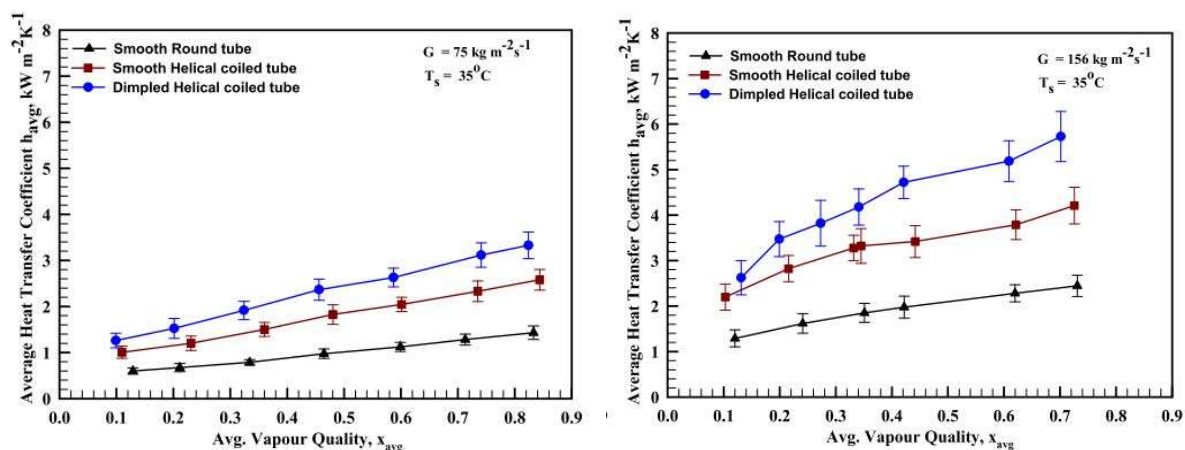
Slika 14. Usporedba koeficijenta prolaza topline za ravne i spiralne cijevi [26].
