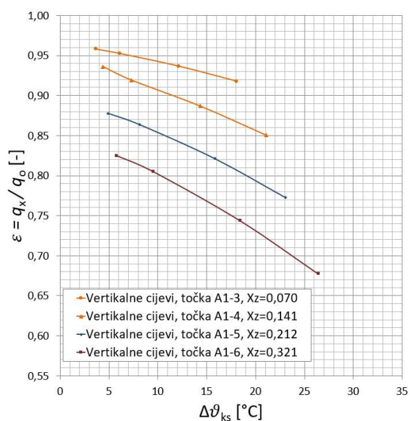
Slika 44. Ovisnost parametra \varepsilon o temp. potencijalu u setu usp. točaka A1 (vertikalne cijevi)
