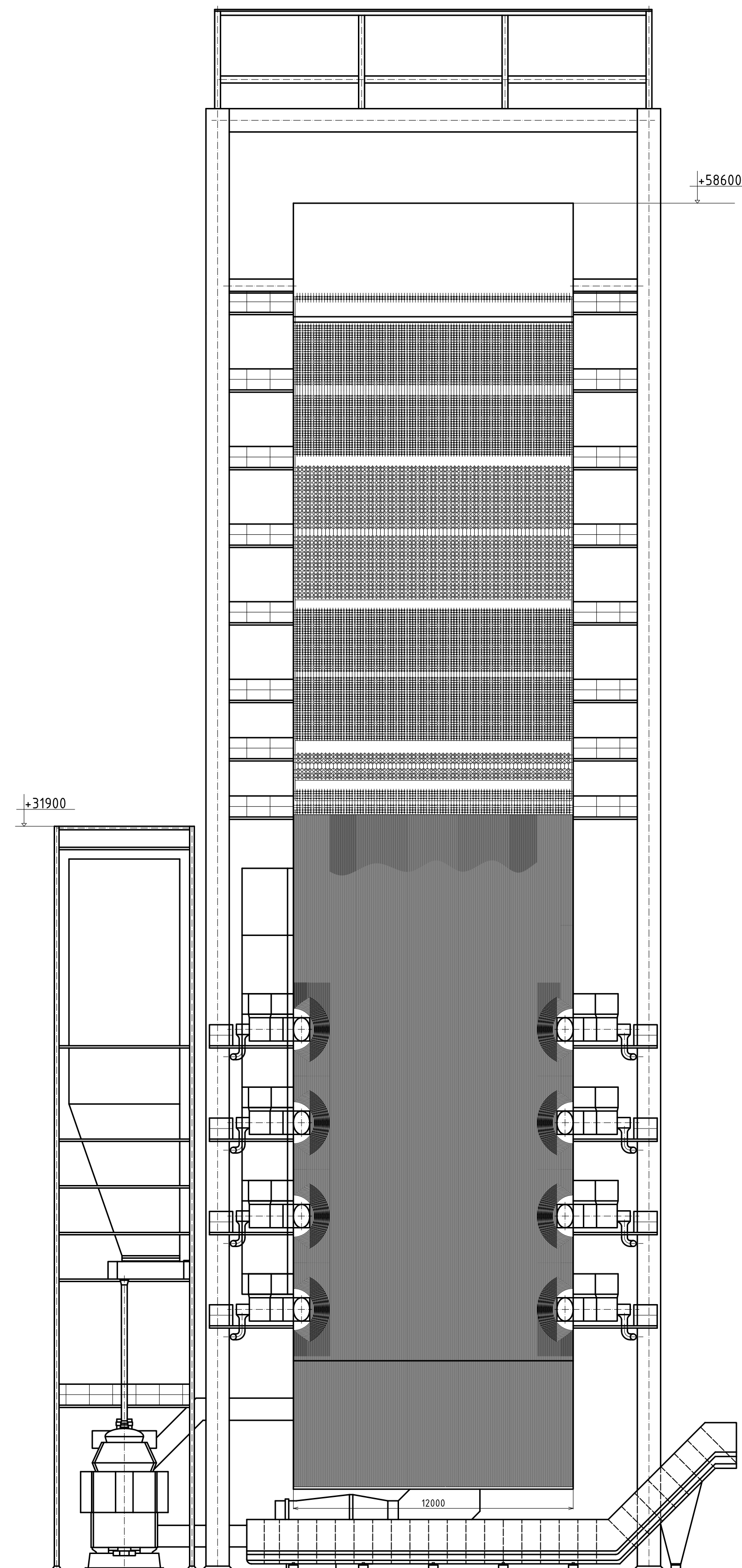
Presjek A-A
