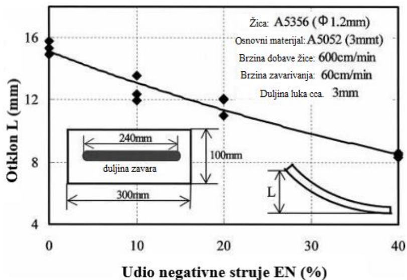
Slika 35. Utjecaj EN omjera na deformaciju otklona kod zavarivanja ploče aluminija debljine 3 mm [3]
