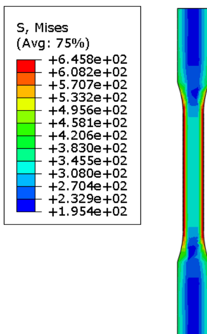
Slika 7.2. Raspodjela ekvivalentnog napreznja prije loma za monotono opterećeni 2D ispitni uzorak
