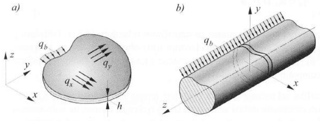
Slika 4.2. a) ravninsko stanje napreznja; b) ravninsko stanje deformacije [25]
