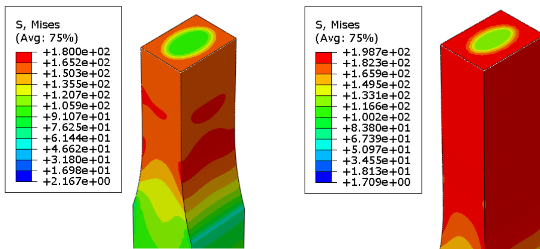
Slika 7.8. Raspodjela ekvivalentnog naprezanja u ciklički opterećenom 3D modelu ispitnog uzorka za dubinu densifikacije d = 0,5 mm (lijevo) i d = 1 mm (desno)
