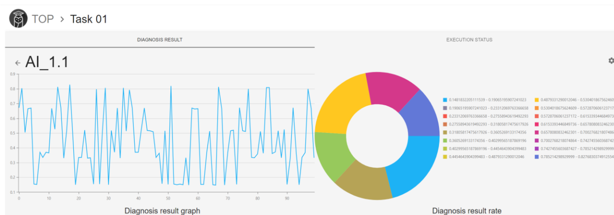
Slika 49. Rezultati dijagnoze
