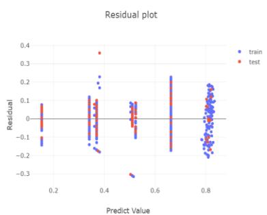
Slika 41. Random Forest
