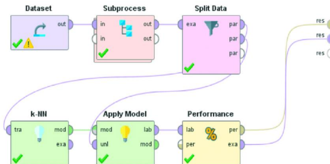
Slika 9. Prikaz procesa u RapidMiner-u [20]
