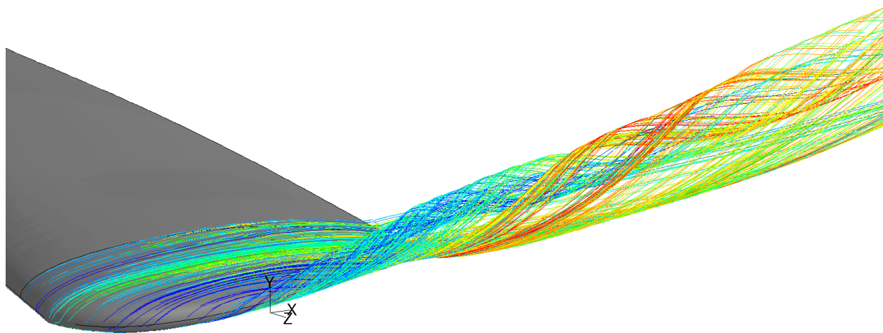
Slika 8.11 Prikaz vrtloženja na vrhu lopatice
