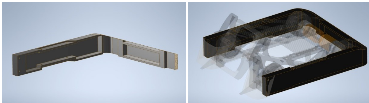
Slika 55. Eggsecutionerov_V3 CAD potrošnog oklopa (lijevo) na sklopu (desno)
