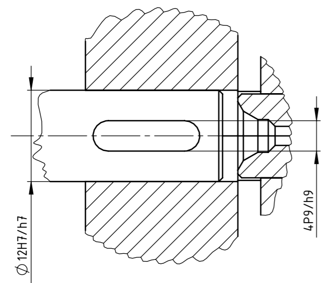
Detalj Z Mjerilo M2:1
