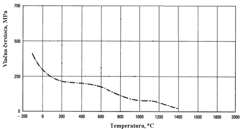
Slika 2. Temperaturna ovisnost vlačne čvrstoće niobija [4]
