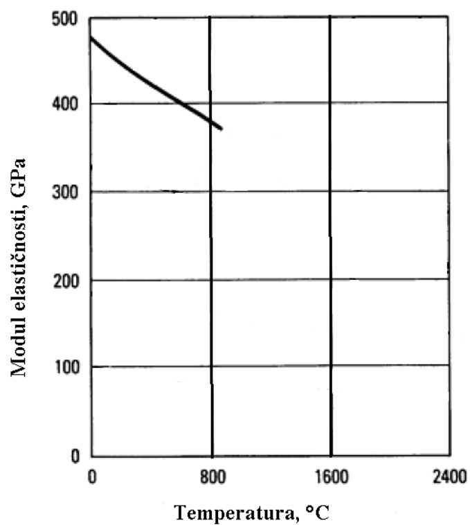
Slika 21. Temperaturna ovisnost modula elastičnosti renija [4]
