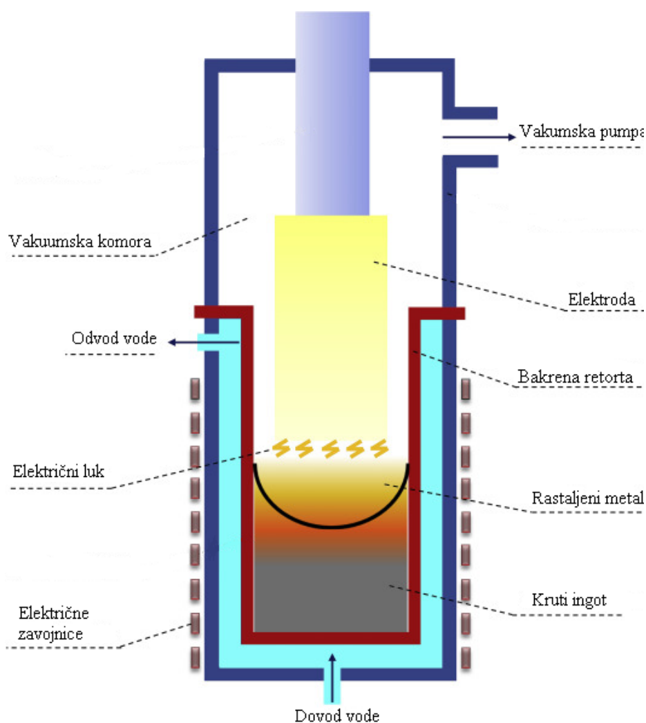
Slika 22. Komora za VAR/VAC tehnologiju [37]
