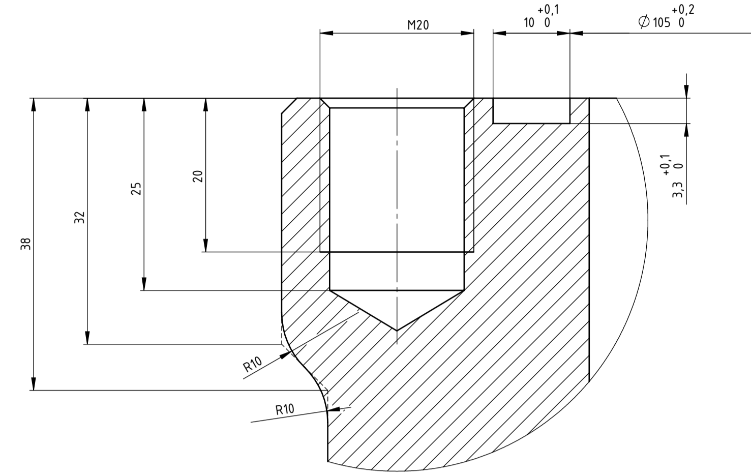
Presjek B-B (2:1)
