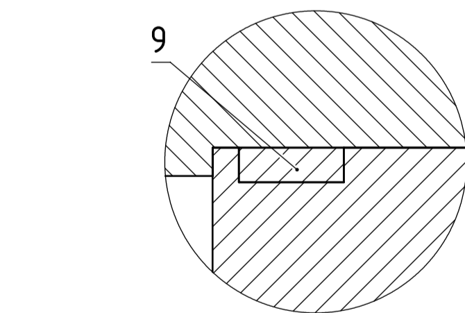
Detalj B (2:1)
