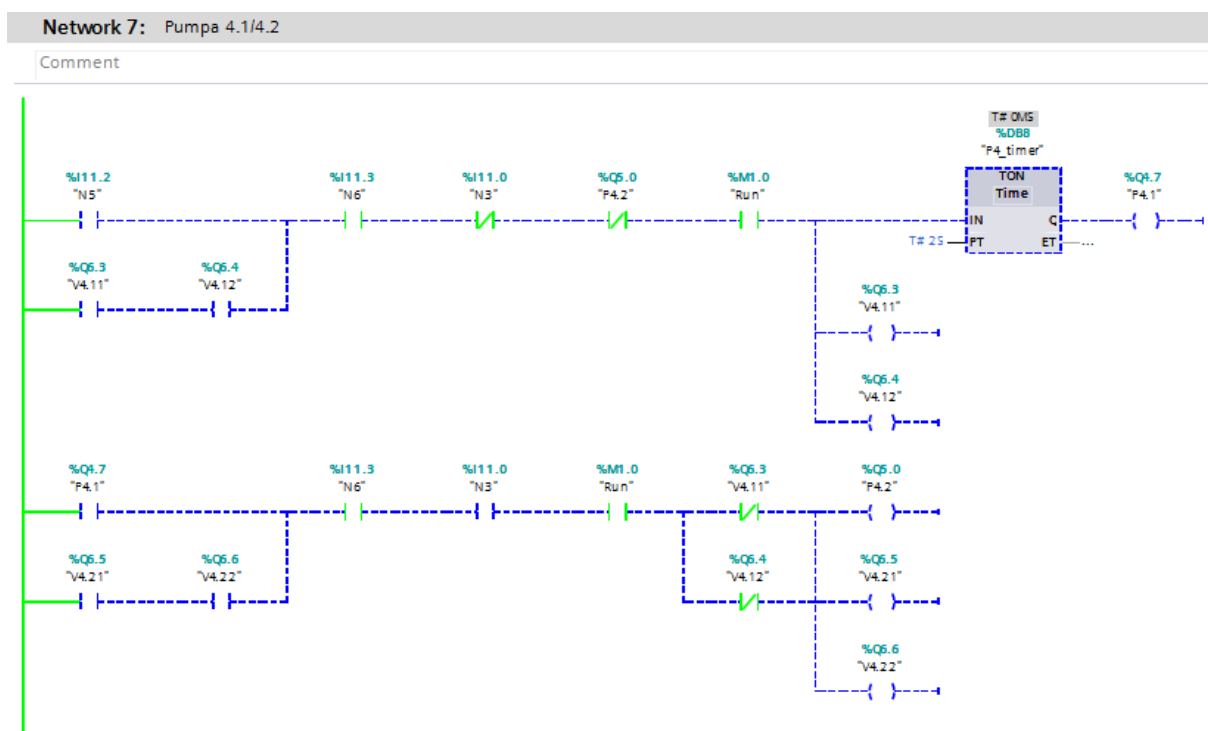
Slika 20. Pumpa P4
