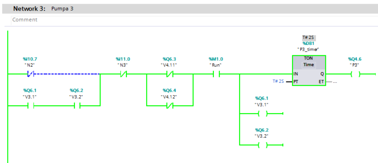
Slika 19. Pumpa P3
