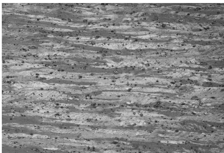
Slika 2. Deformacijom izdužena kristalna zrna tehnički čistog aluminijsa
