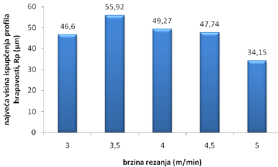
Slika 3.34. Prikaz ovisnosti najveće visine ispuščenja profila hrapavosti o brzini rezanja – Al legura – plazmeni plin zrak
