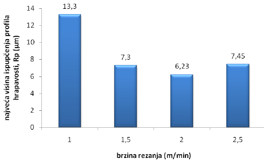
Slika 3.9. Prikaz ovisnosti najveće visine ispućenja profila hrapavosti o brzini rezanja – nelegirani čelik – plazmeni plin zrak
