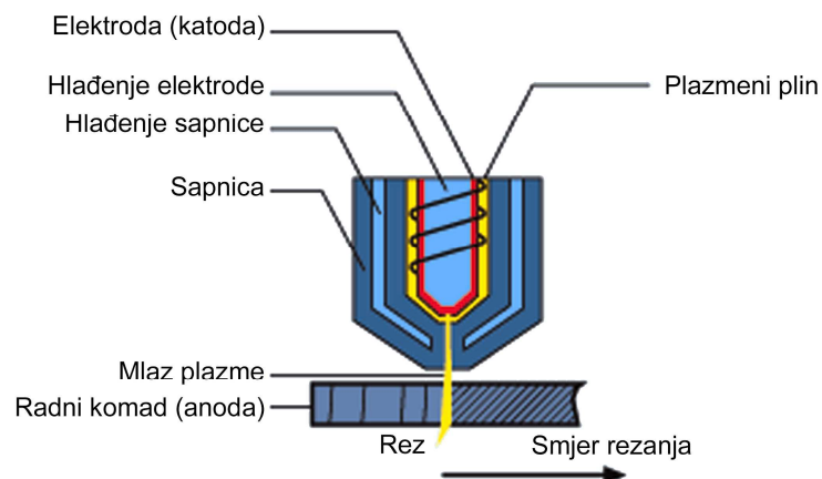
Slika 2.2. Standardni postupak plazma rezanja [2]
