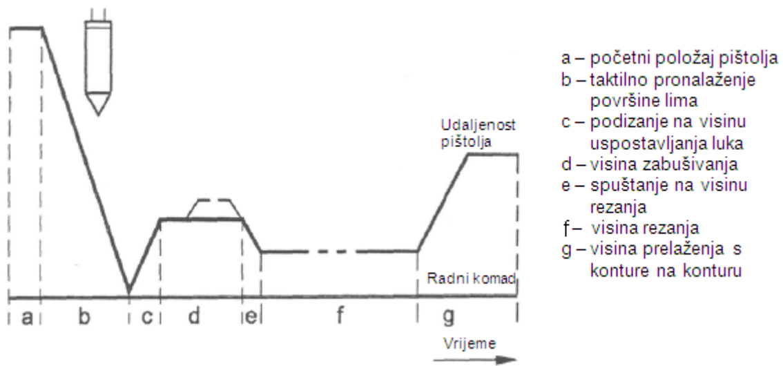
Slika 2.12. Tijek gibanja pištolja kod CNC upravljano rezanja plazmom [9]
