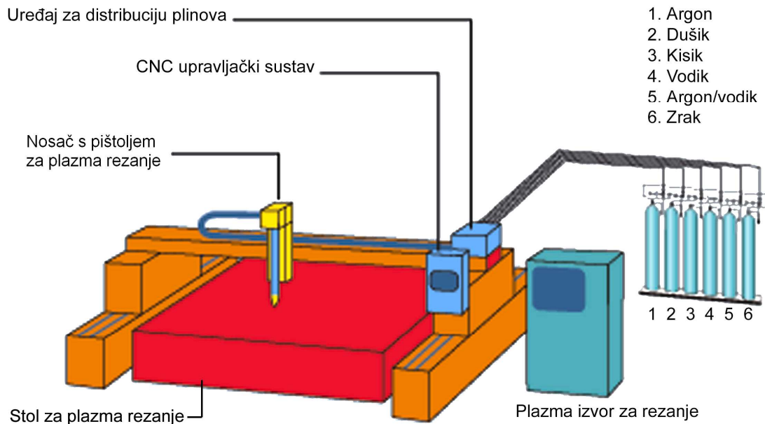
Slika 2.8. Sustav strojnog plazma rezanja [2]
