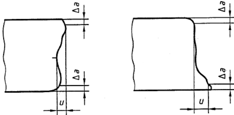
Slika 2.19. Tolerancija okomitosti ili kutnosti [20]
