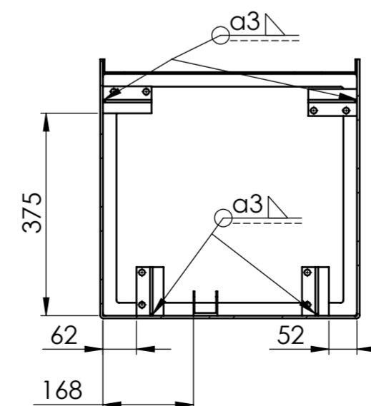
PRESJEK C-C
