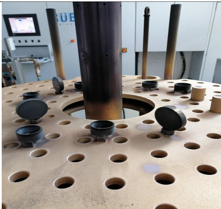
Slika 24. Prstenovi nakon nitiranja u plazmi
