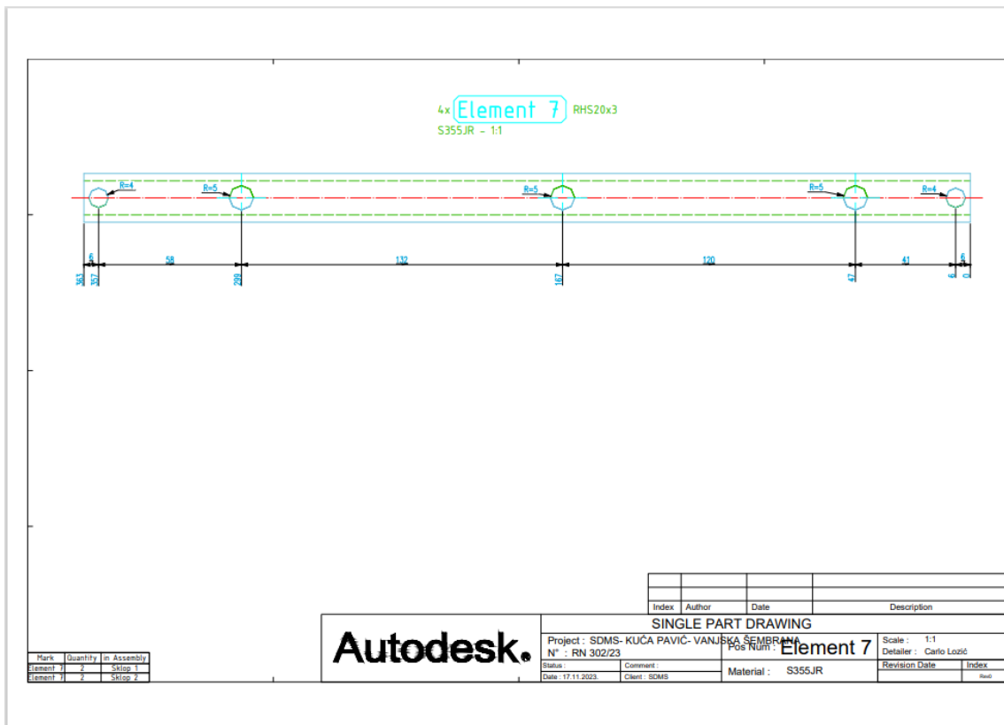
Slika 24. Prikaz radioničkog nacrt 2/2
