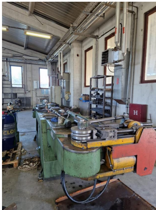
Slika 22. Savijačica na trn
