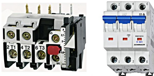
Slika 77. Bimetalna zaštita [23] i osigurač [24]
