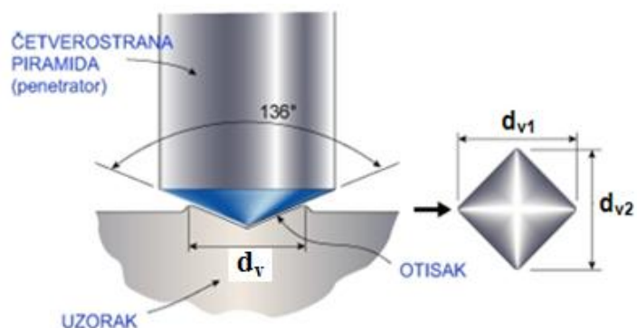
Slika 13. Utiskivanje Vickersovog indentora i izgled otiska [13]
