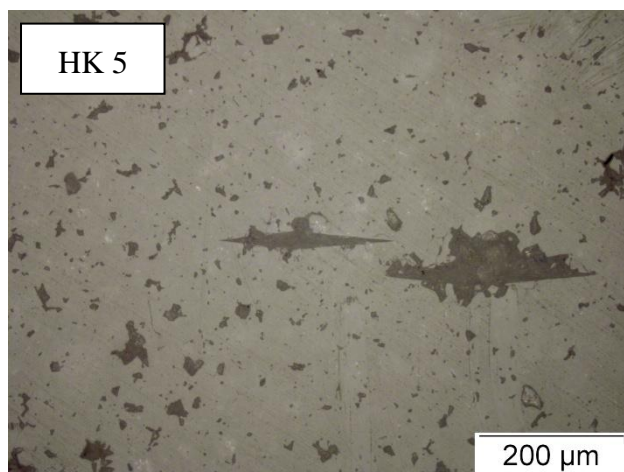
Slika 49. Otisci Knoopovog indentora na površini brušenoj SiC papirom znatosti 4000
