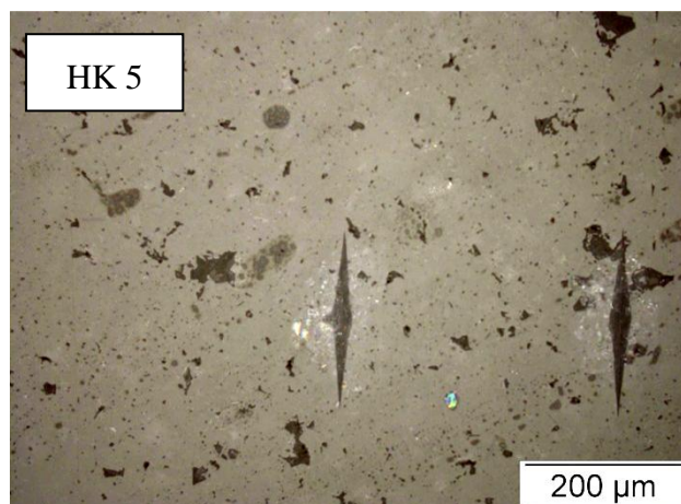
Slika 51. Otisci Knoopovog indentora na površini poliranoj dijamantnom pastom veličine abraziva 1 μm
