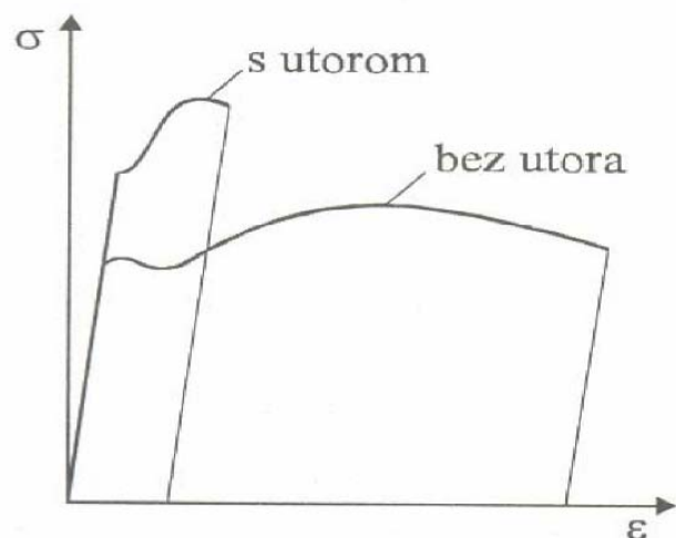
Slika 2.5 Dijagram naprezanje-istezanje
