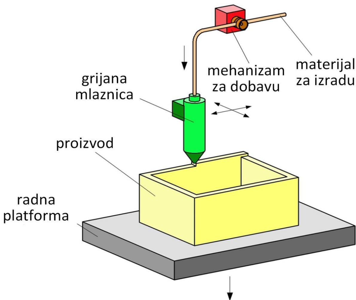
Slika 34. FDM postupak [23]
