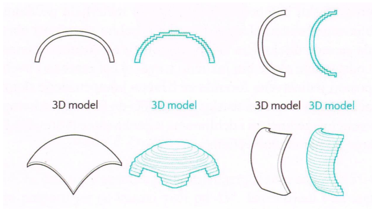
Slika 20. Prikaz pravilne orijentacije modela prilikom 3D ispisa [23]
