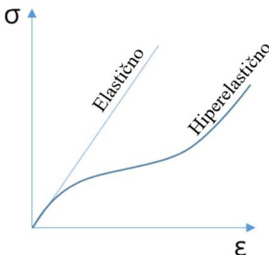
Slika 17. Krivulje naprezanja-deformacija za elastične i hiperelastične materijale [49]
