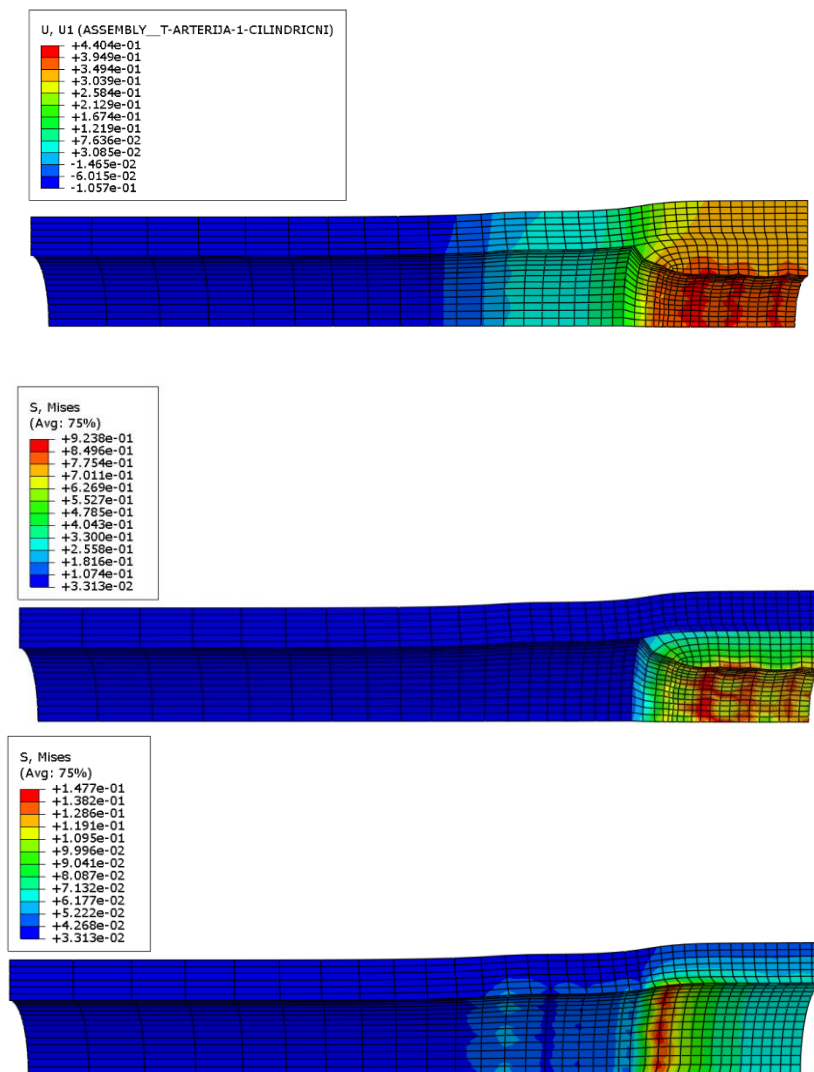
Slika 39. Pomaci [mm] i naprezanja [N/mm 2 ] za četvrti set parametara i Favus stent
