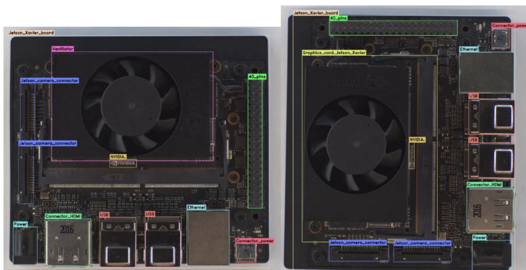
Slika 24. Detekcije u različitim orijentacijama
