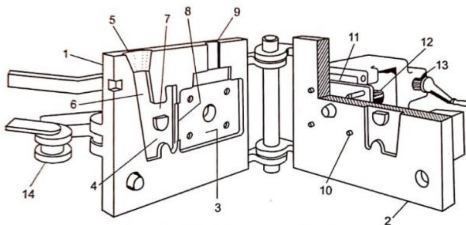
1-pomična ploča kalupa, 2-nepomična ploča, 3-kalupna šupljina, 4-uljevni sustav, 5-čaška, 6-spust 7-razvodnik, 8-ušća, 9-pojilo, 10-jezgra, 11-jezgreća ploča 12-zubna letva za povlačenje jezgri, 13-zupčanik s ručnim pogonom, 14-brava s ekscentrom za zatvaranje kalupa
