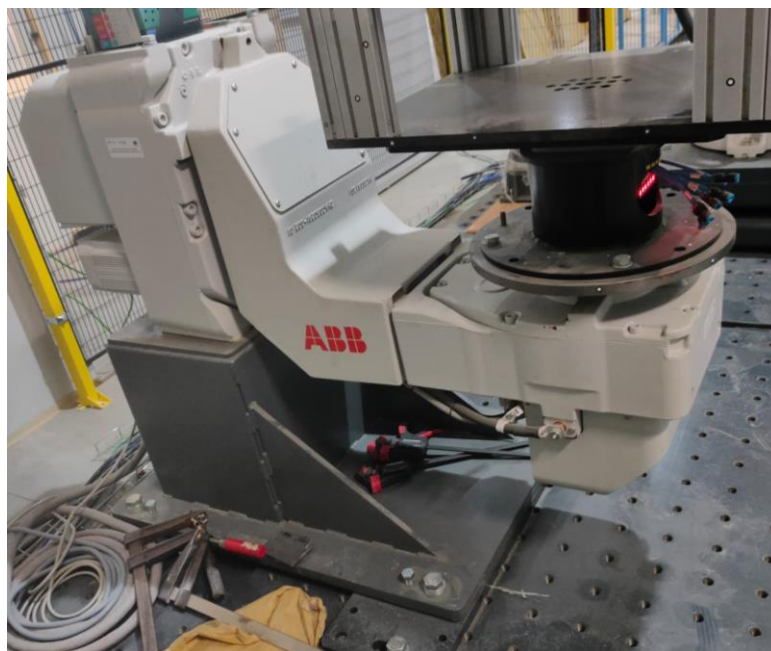
Slika 7. ABB-IRBP-A-500-1000 postavljen u robotskoj obradnoj ćeliji
