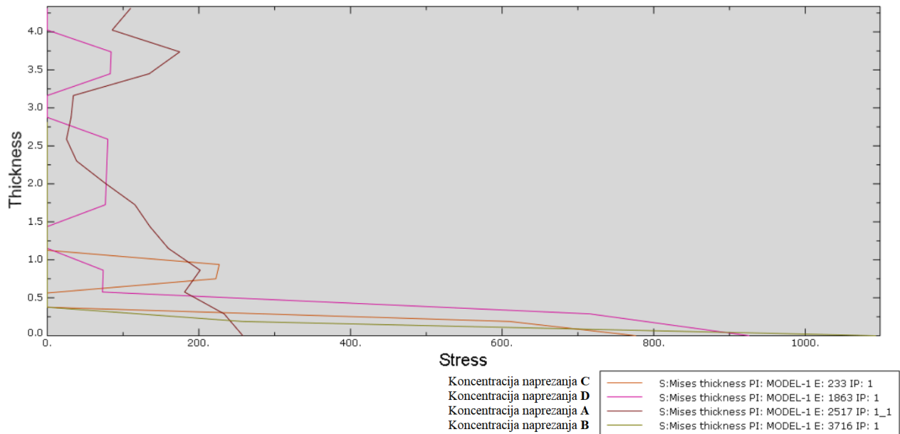
Slika 41. Raspodjela ekvivalentnih von Mises naprezanja [MPa] po debljini [mm] stijenke za prvu kompozitnu konfiguraciju zaštitne konstrukcije
