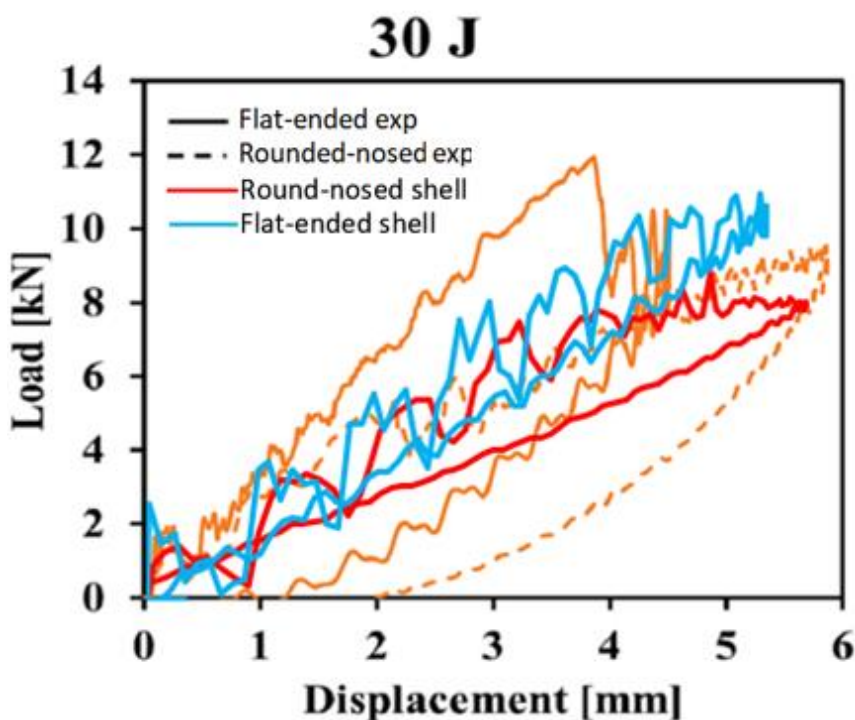
Slika 23. Dijagram ovisnosti kontaktne sile o pomaku za energiju udara 30 J
