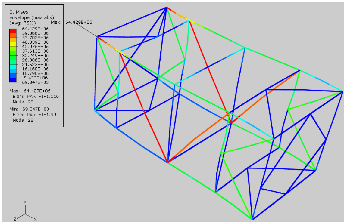
Slika 4.9 Rekonstruirana rešetka - prikaz maksimalnih ekvivalentnih napreznja – djelovanje horizontalne tlačne sile F=75 kN na lijevom kraju
