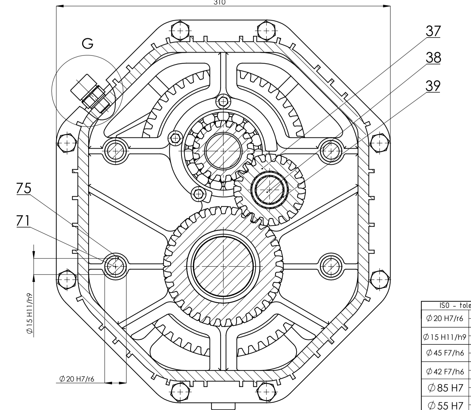
E-E (M 1:2)
