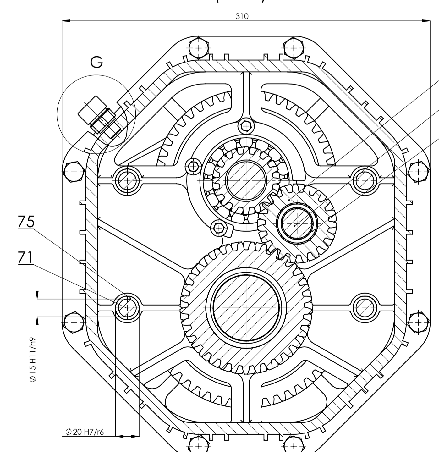
E-E (M 1:2)
