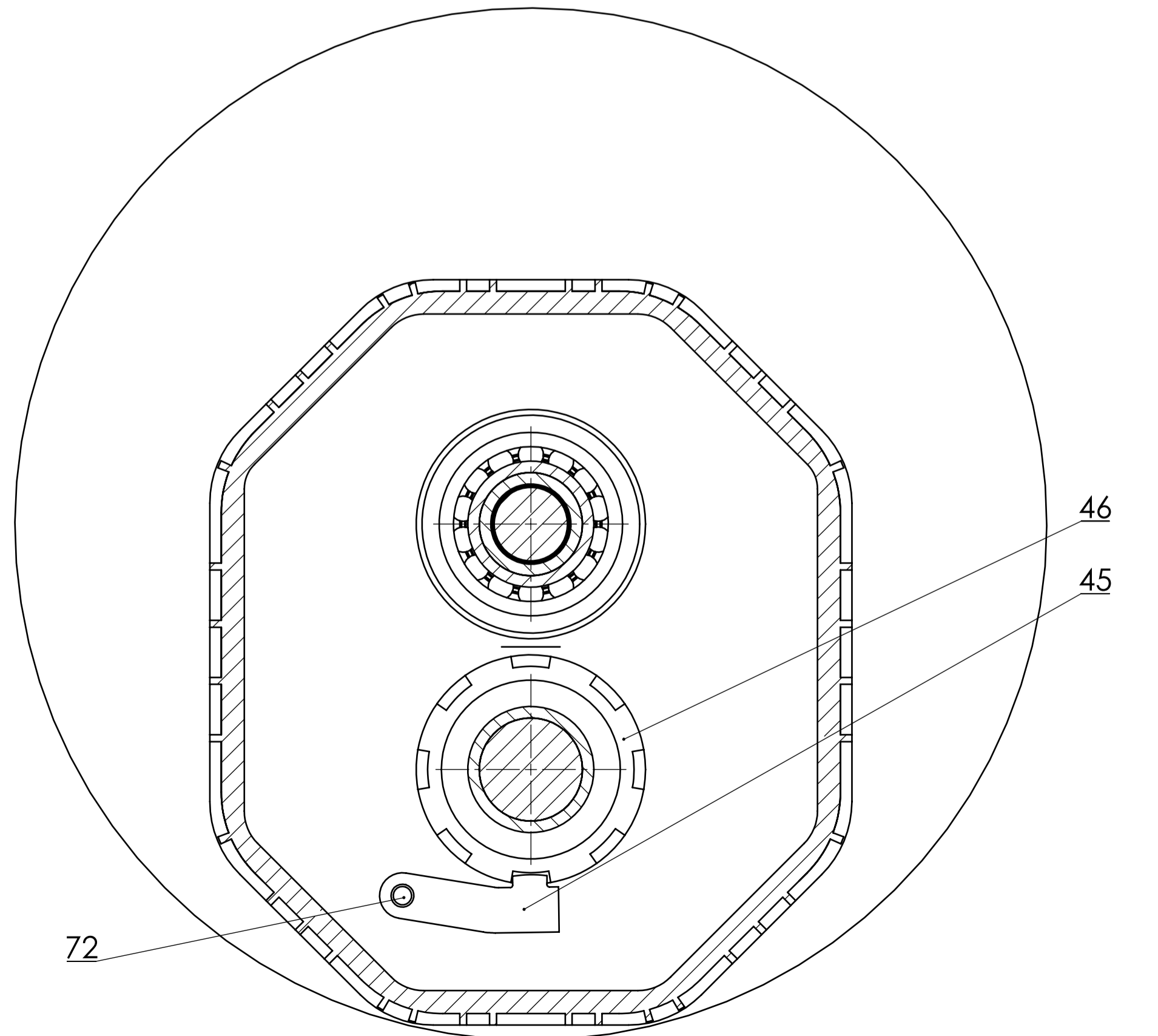
F-F (M 1:2)
