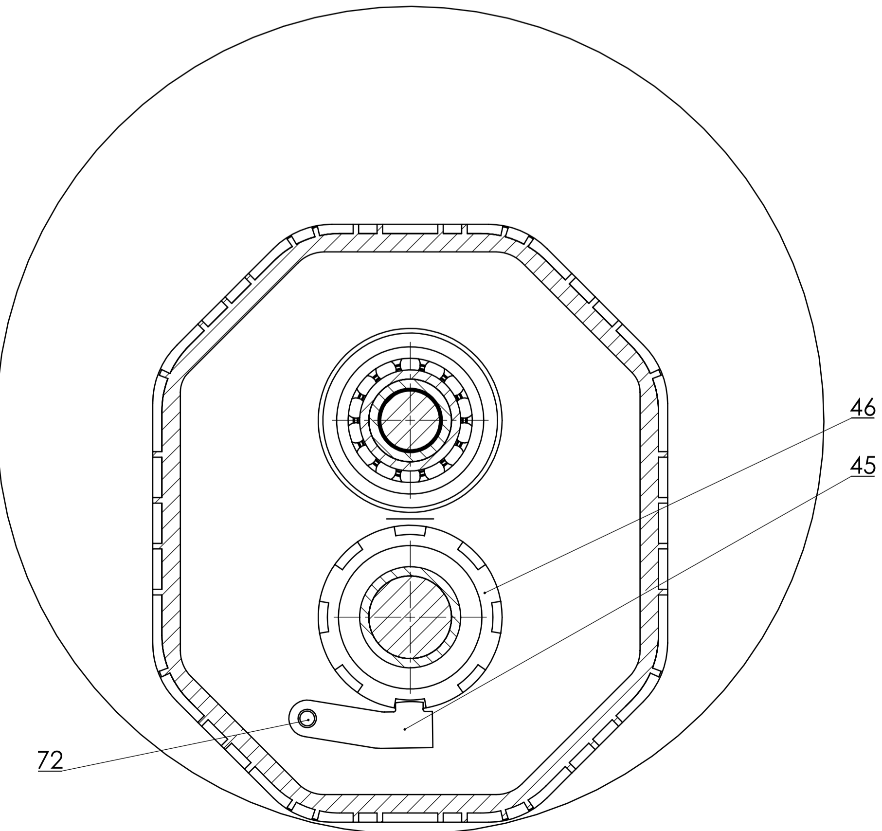
F-F (M 1:2)
