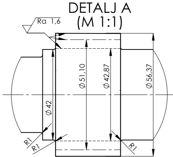
DETALJ A (M 1:1)
