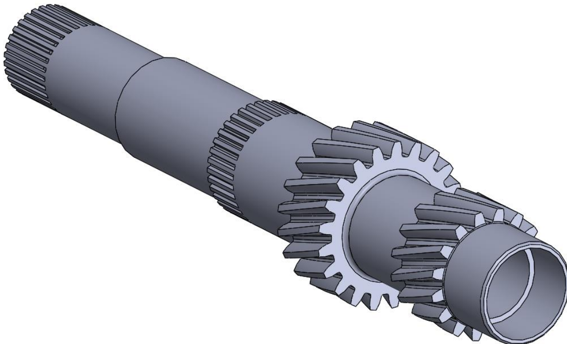
Slika 7.7 Ulazno vratilo V_2
