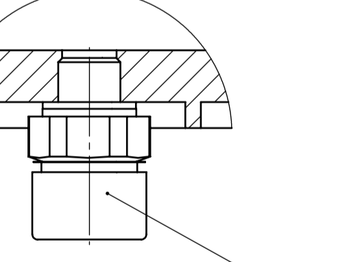
DETALJ C (M 1:1)
