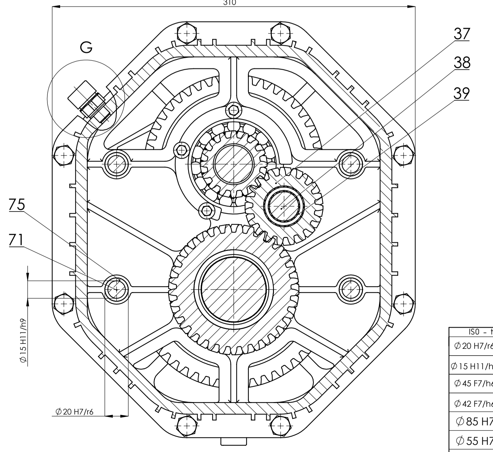
E-E (M 1:2)
