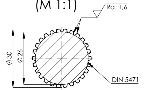
C-C (M 1:1)
