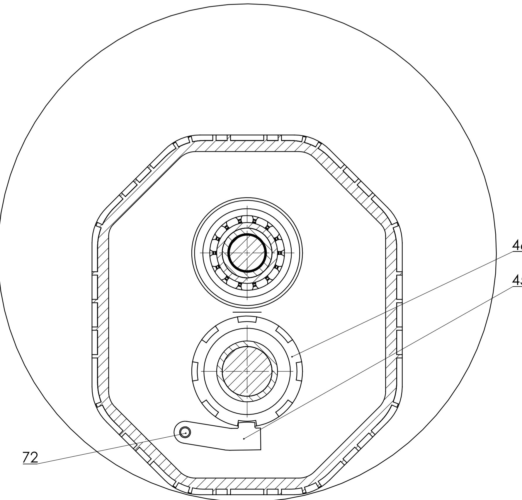
F-F (M 1:2)
