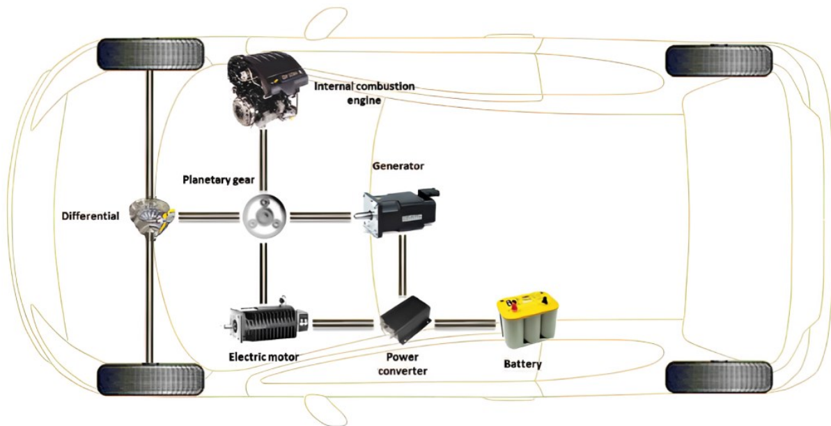
Slika 5. Serijsko-paralelna konfiguracija hibridnog pogona (preuzeto iz [1]).
