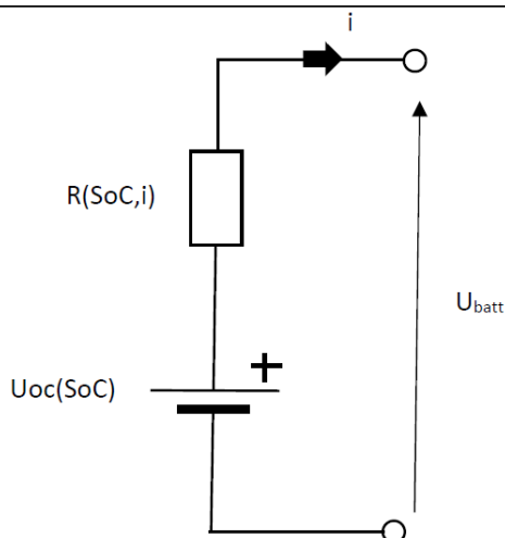
Slika 24. Model baterije zasnovan na nadomjesnom krugu.
