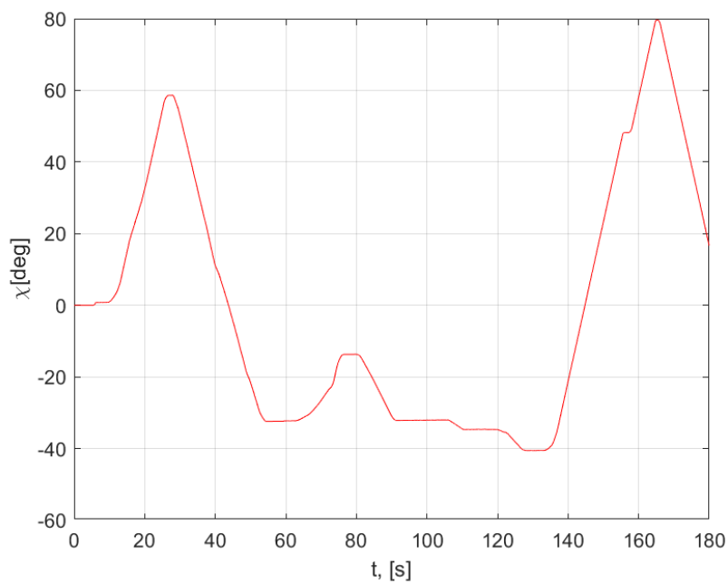
Slika 27: \chi tijekom simulacije s upravljanjem u realnom vremenu
